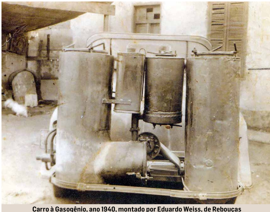
Carro à Gasogênio, ano 1940, montado por Eduardo Weiss, de Rebouças
